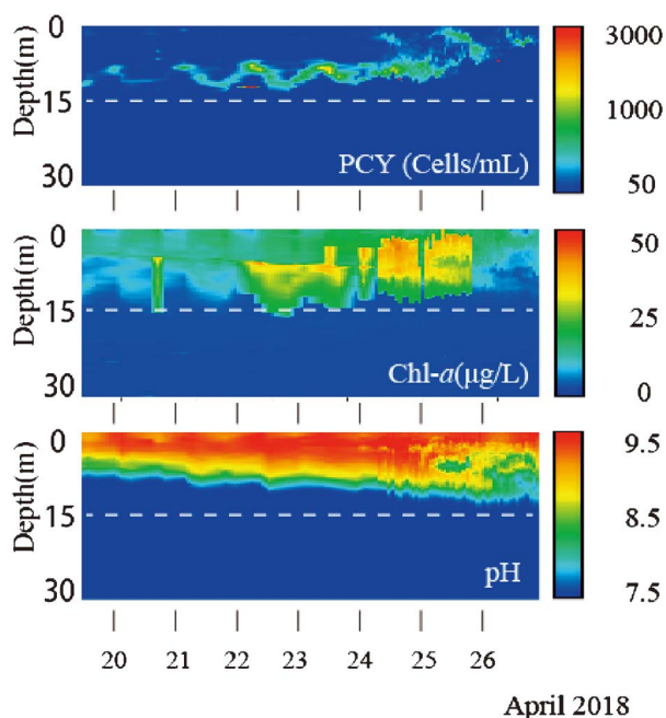
図4 貯水池におけるラン藻類の増殖過程
