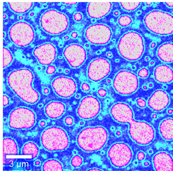
図3 PMMA/SBR ブレンドの海島構造。PMMA が赤色、SBR が青色。(WITec 社よりデータ提供)
