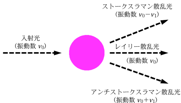
図1 レイリー散乱とラマン散乱
