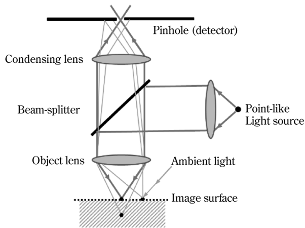
図2 共焦点レーザー顕微鏡の概略図
