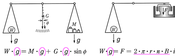
図1 機械式天びんと電磁式天びんの機構 (図中右： 2 \cdot \pi \cdot r \cdot n ：コイルの長さ（ r ：半径， n ：巻き数）， B ：磁束密度， i ：電流）
